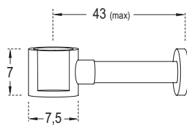
S7 Reduced shape siphon. Chrome. Siphon réduit. Chrome.
