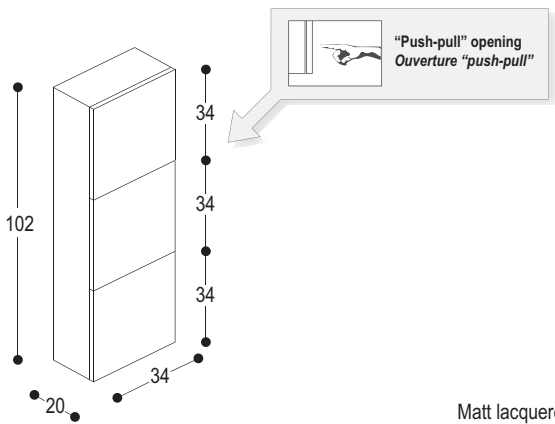
BQ3 Wall unit with 3 left or right doors. Two shelves. Armoire murale avec 3 portes droite ou gauche. Deux étagères.
