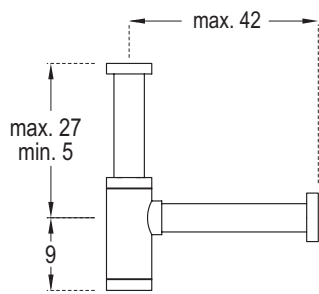
S3 Bottle siphon. Siphon bouteille.
