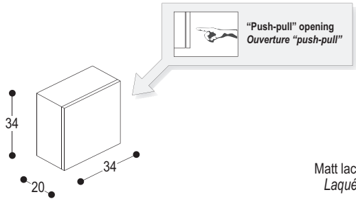
BQ1 Wall unit with 1 left or right door. Armoire murale avec 1 porte droite ou gauche.
